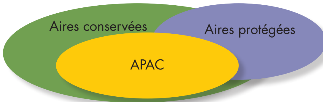
Schéma 3. Superposition incomplète des aires protégées, des aires conservées et des APAC
