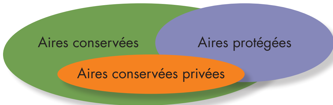
Schéma 2. Superposition incomplète des aires protégées, des aires conservées et des aires conservées privées
