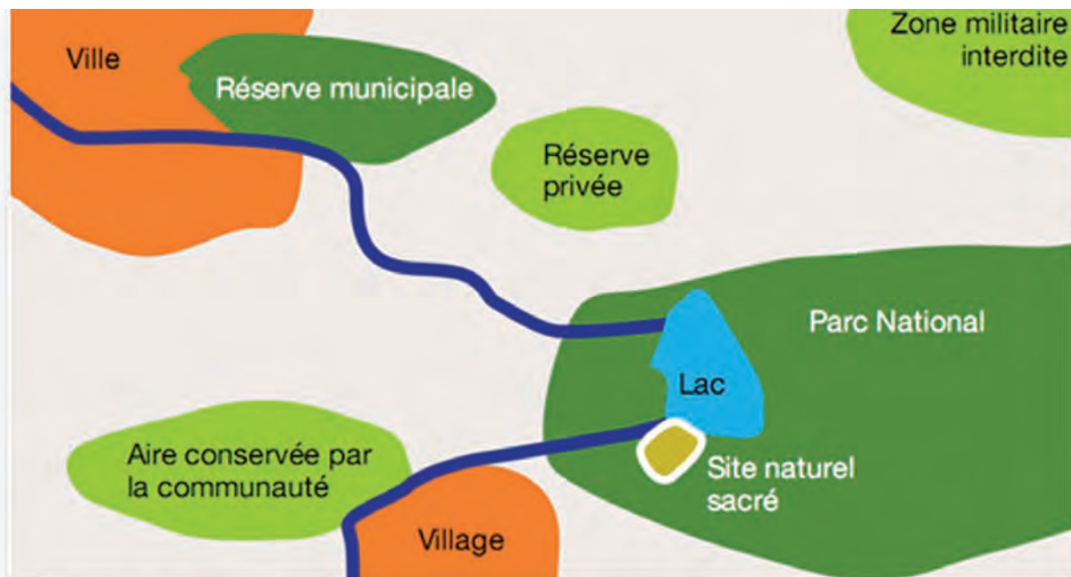
Schéma 4. Diverses mesures spatiales de conservation par aire et territoire dans le paysage
